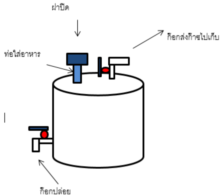
ถังที่ 1 ถังหมักก๊าซ
